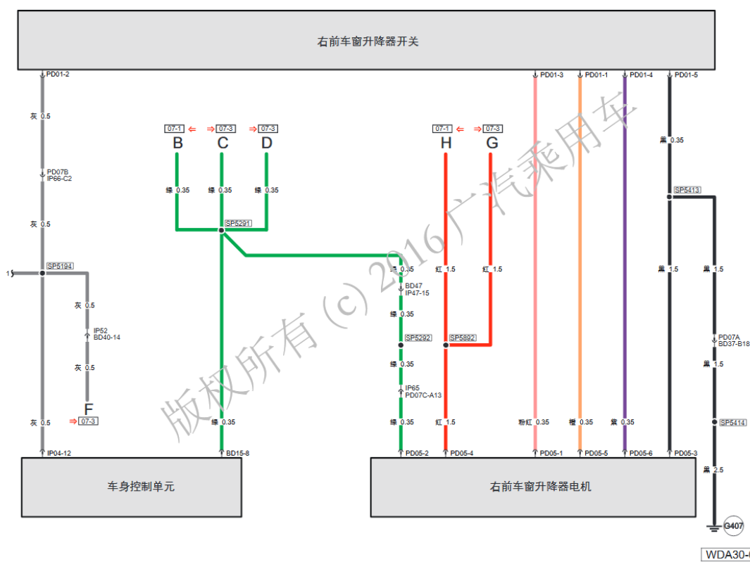
07-2 电动车窗升降电路图
